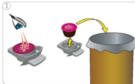
1 Stop met de bereiding, trek de capsulehouder uit de machine en controleer de capsule. Er mag maar één gaatje in de capsule zitten. Gooi een capsule met meer dan één gaatje weg.
